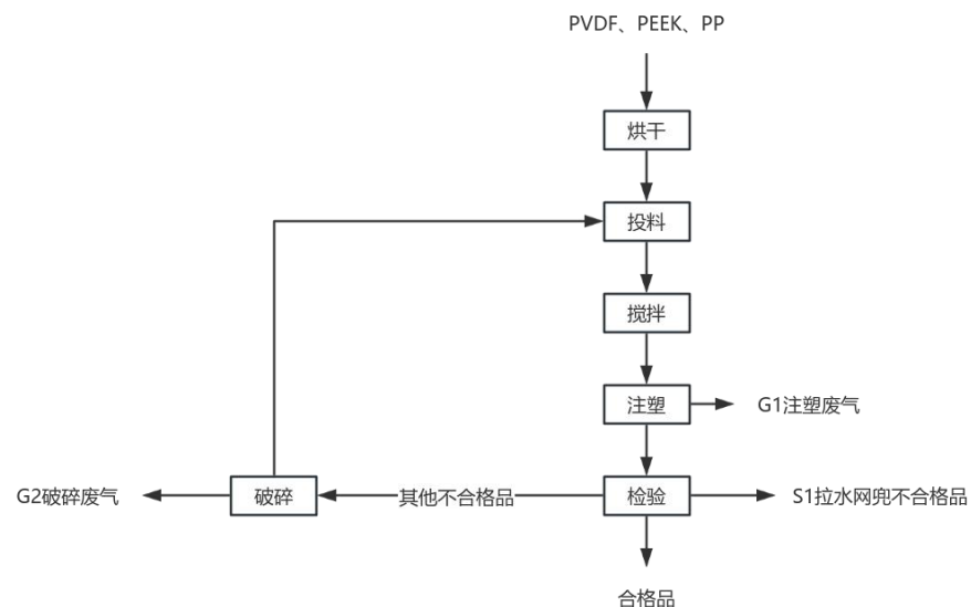
图 2-2 注塑件生产工艺流程图
